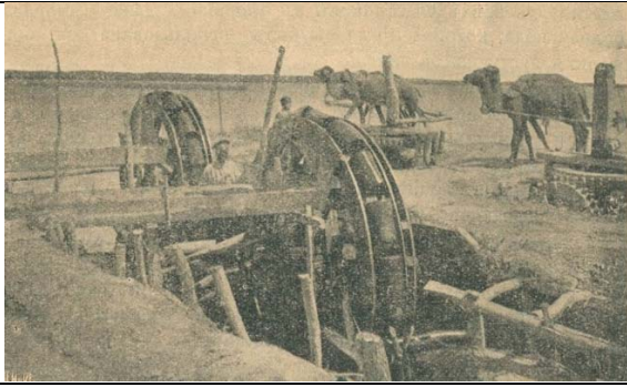
Рис. 3 – Верблюжий чигирь (приведение в движение чигиря с помощью верблюда). Правобережье Сырдарьи. Конец XIX в. Снимок М.Дьякова [2, с.19].
