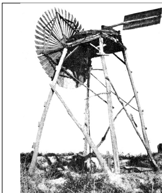
Рис. 1 – Ветряной чигирь (поливная установка, работающая на ветру), Перовский уезд, 1910 год, октябрь [4].
